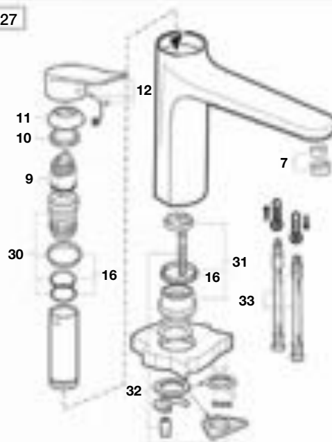
Grifería para cocina
