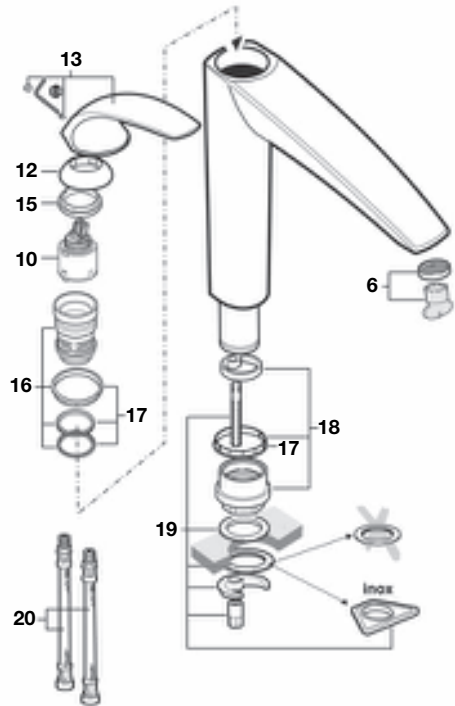
Grifería para cocina
