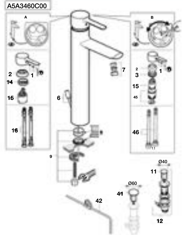
Grifería de caño alto para lavabo
