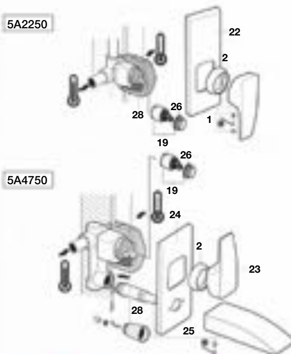
Grifería para baño o ducha y para lavabo
