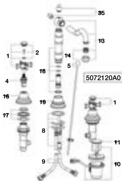
Grifería para lavabo
