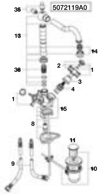
Grifería para baño y ducha
