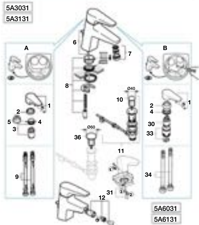
Grifería para baño y ducha
