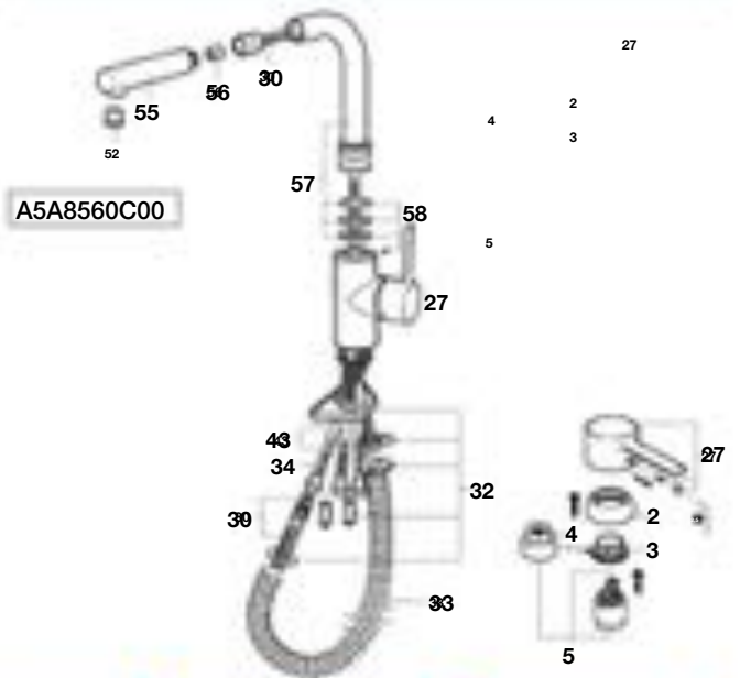
Grifería para cocina
