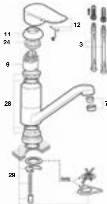
Grifería para cocina
