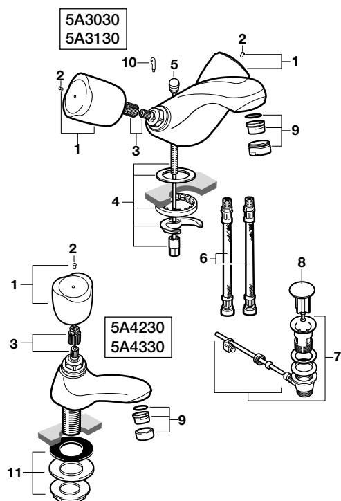
Grifería para bidé
