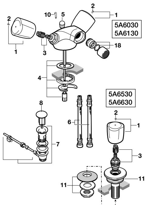
Grifería para bidé
