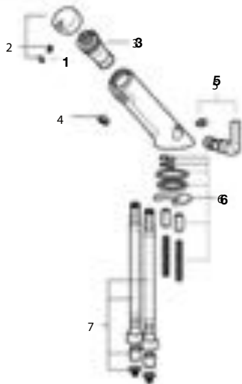
Mezclador de repisa para lavabo
