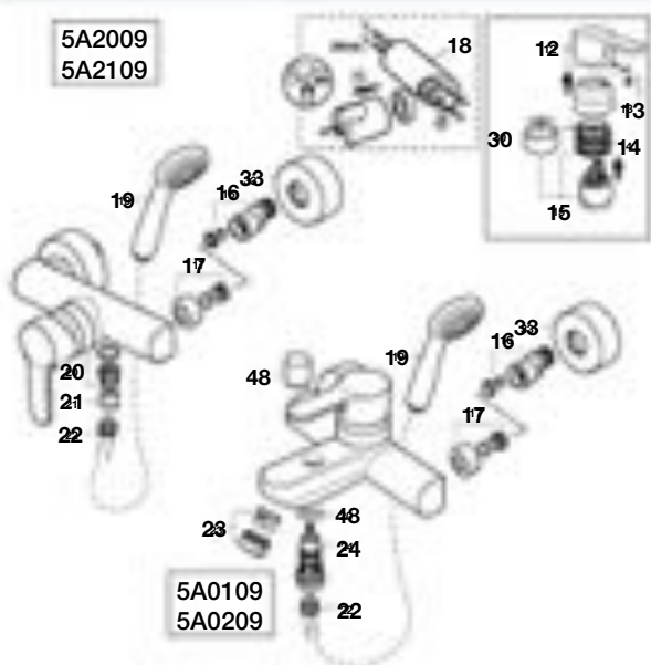
Grifería para baño y ducha
