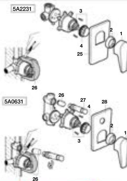
Grifería empotrable para baño y ducha
