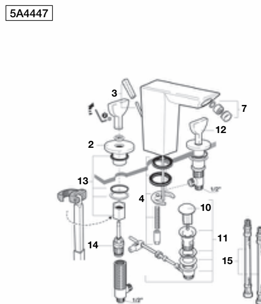
Grifería bimando para lavabo
