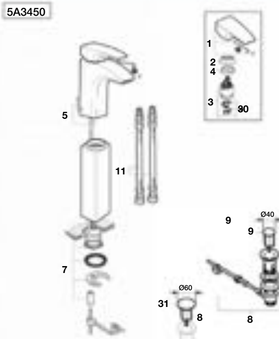
Grifería de caño alto para lavabo
