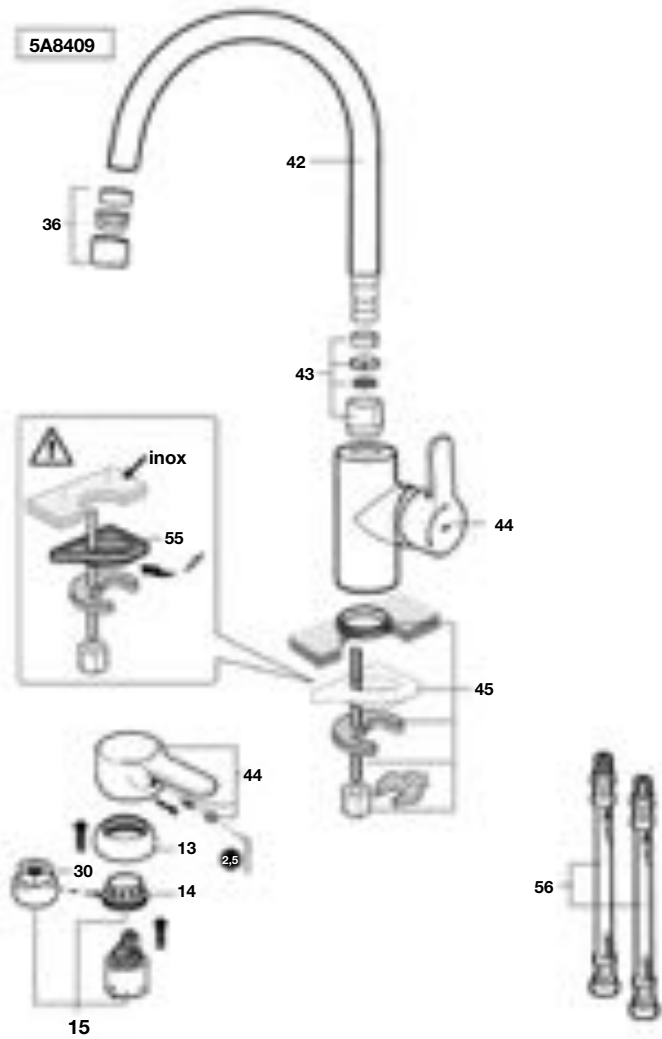
Grifería para cocina
