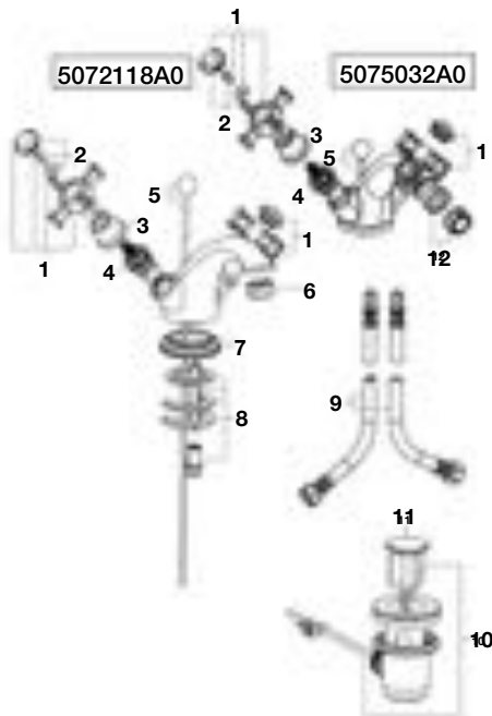
Grifería para lavabo y bidé
