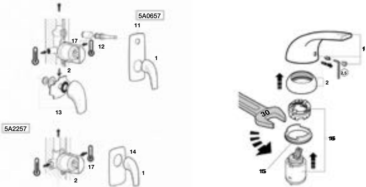
Grifería empotrable para baño y ducha
