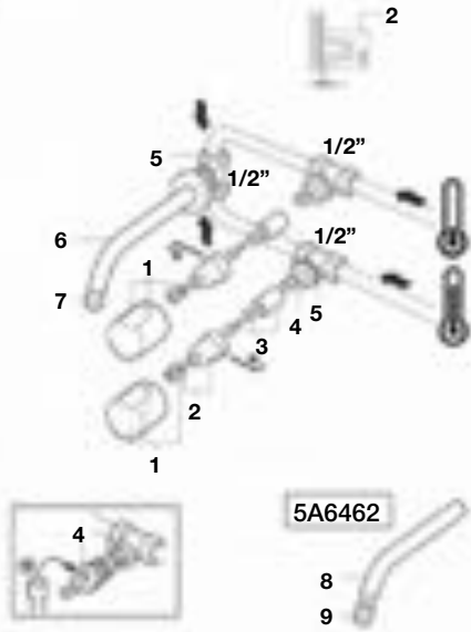
Grifería para lavabo y bidé
