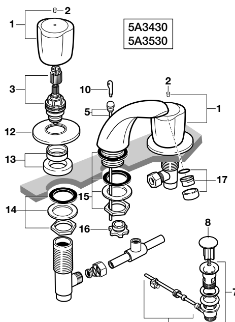
Grifería para lavabo
