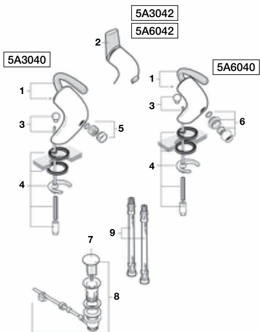
Grifería para lavabo y bidé
