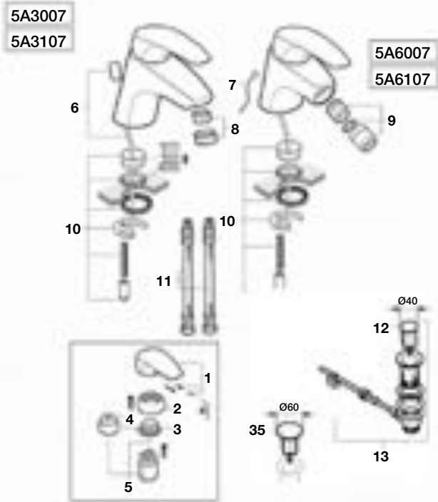
Grifería para lavabo y bidé
