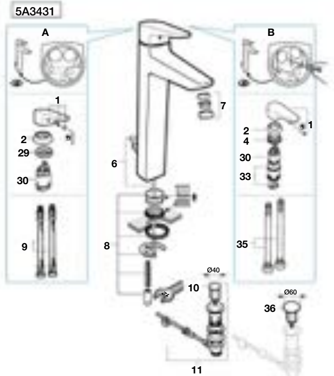
Grifería de caño alto para lavabo
