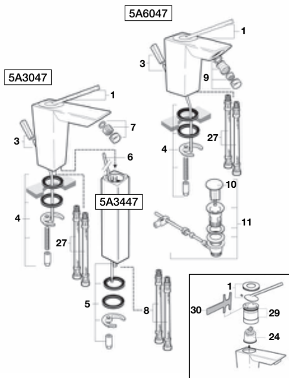
Grifería empotrable para lavabo
