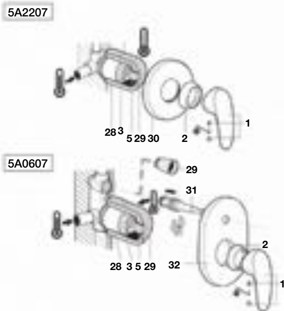
Grifería empotrable para baño y ducha
