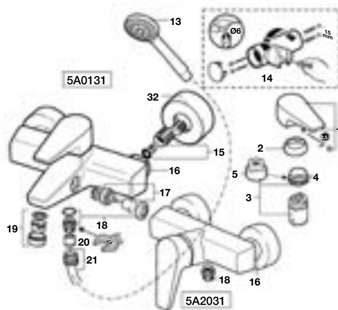
Grifería para baño y ducha
