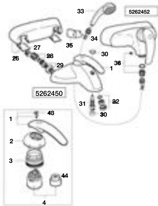
Grifería para baño y ducha
