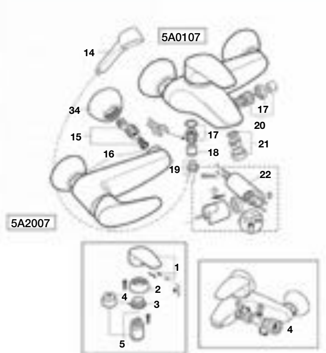
Grifería para baño y ducha
