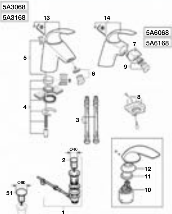
Grifería para lavabo y bidé
