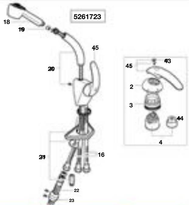
Grifería para cocina
