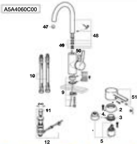
Grifería para lavabo
