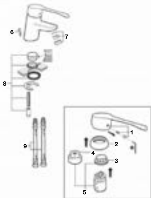
Grifería para lavabo
