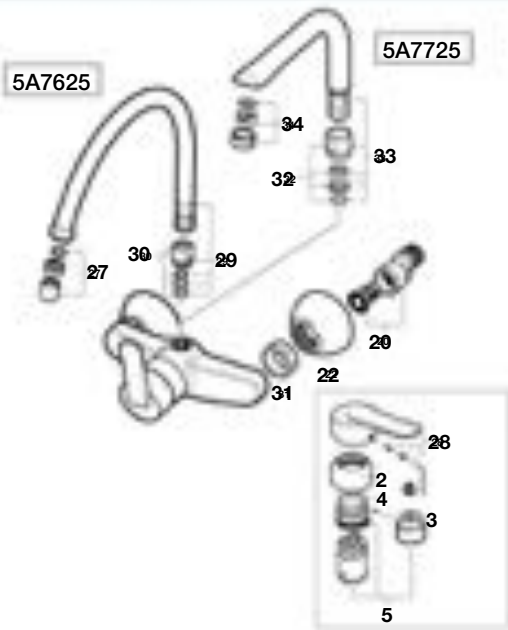
Grifería para cocina
