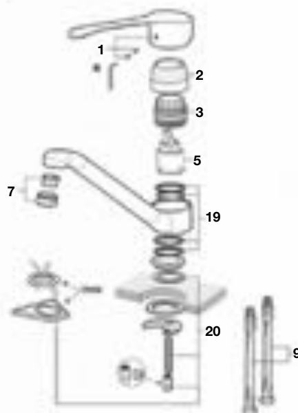
Grifería para cocina
