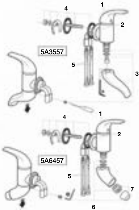
Grifería empotrable para baño y ducha
