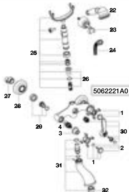
Grifería para baño y ducha
