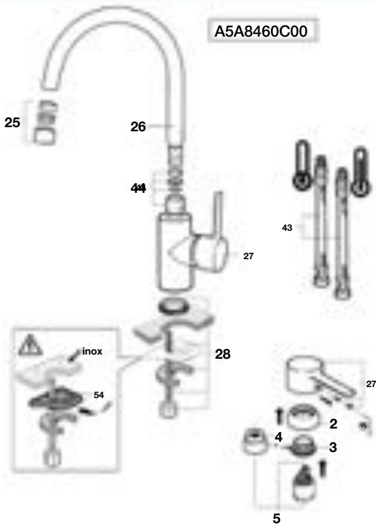
Grifería para cocina
