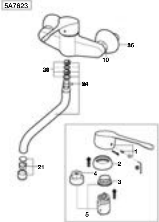
Grifería para cocina
