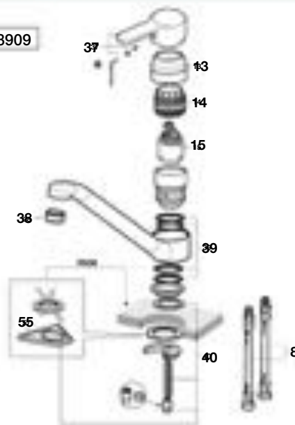
Grifería para cocina
