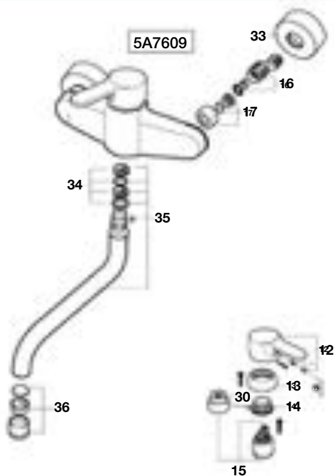
Grifería para cocina
