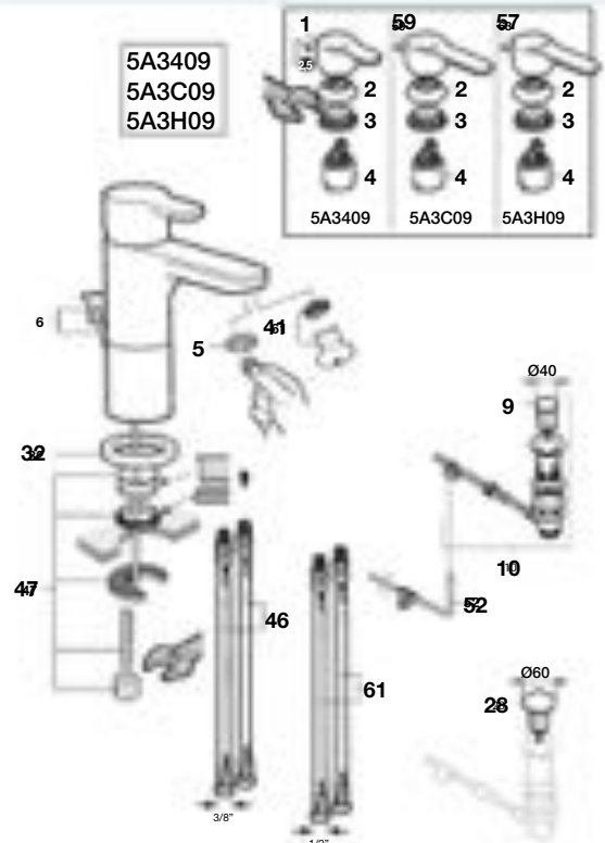
Grifería para lavabo
