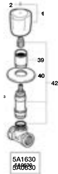
Llaves de paso de 3/4"
